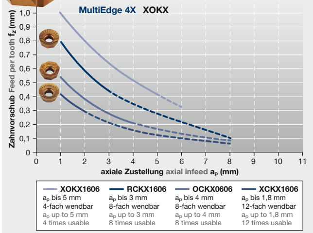
Zahnvorschub des MultiEdge 4X verglichen mit anderen Plattenausführungen Feed per tooth of MultiEdge 4X compared with other inserts shape
